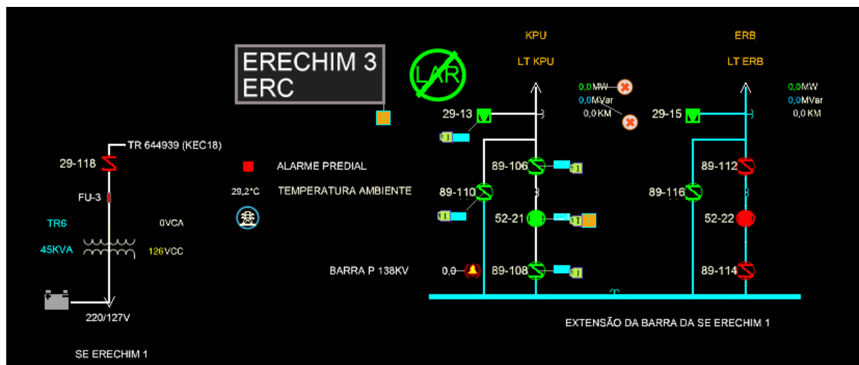
Figura 3 – Diagrama Unifilar da Subestação Erechim ERC
