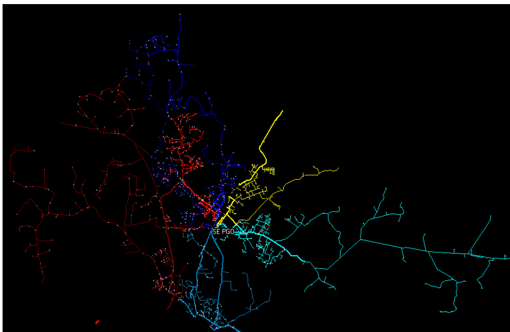
Figura 14 - Mapa Geométrico da subestação Salto 1 – Porto Góes (PGO)
