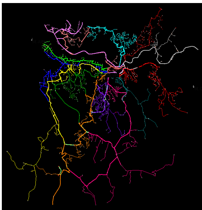
Figura 23 - Mapa Geométrico da subestação Várzea Paulista (VPL)
