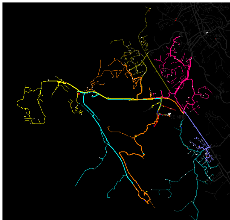
Figura 12 - Mapa Geométrico da subestação Vinhedo 2 – Marambaia (MRB)
