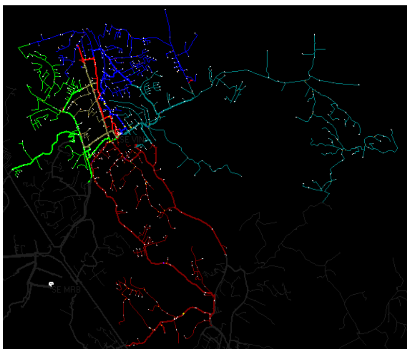
Figura 21 - Mapa Geométrico da subestação Vinhedo 1 (VIN)
