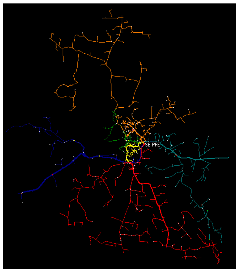
Figura 13 - Mapa Geométrico da subestação Porto Feliz (PFE)
