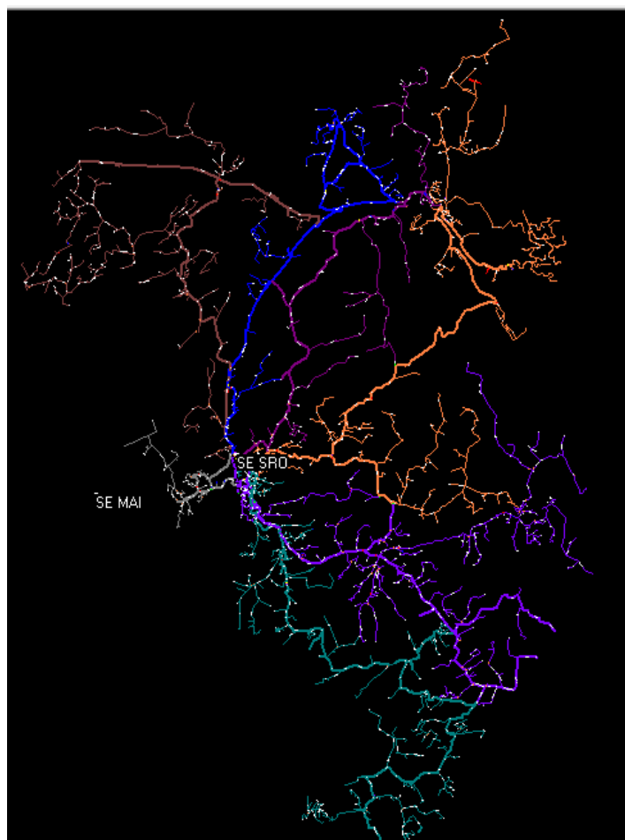
Figura 20 - Mapa Geométrico da subestação São Roque (SRO)
