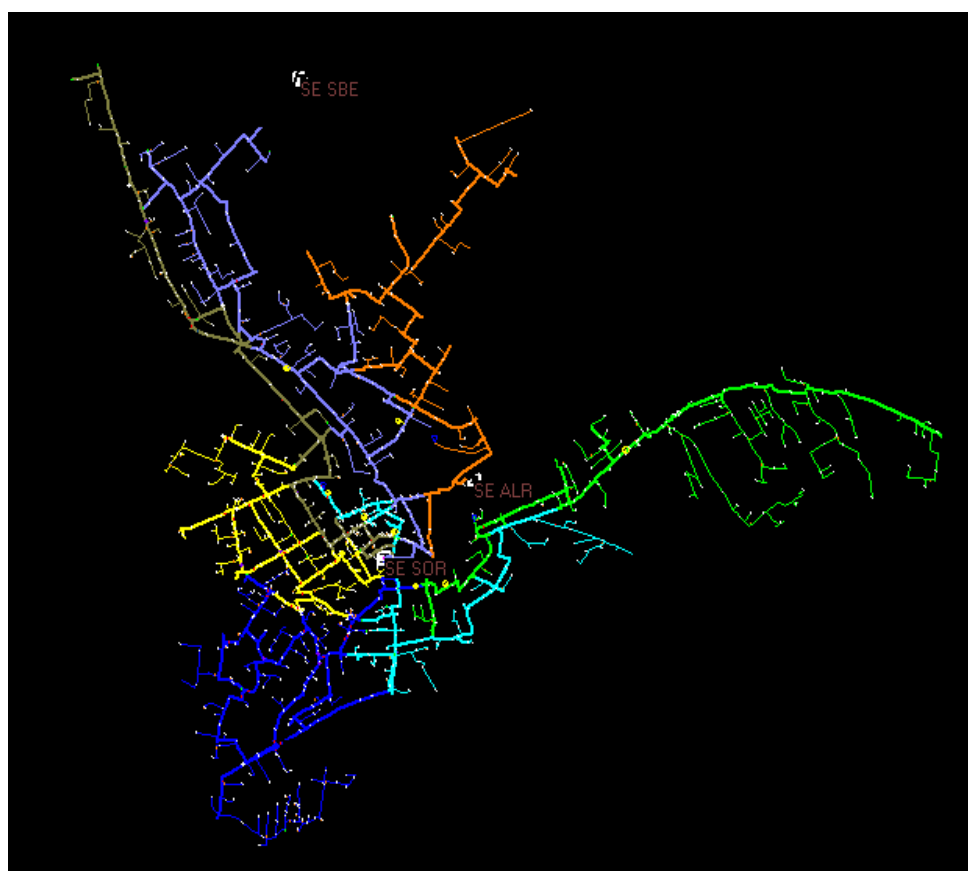
Figura 19 - Mapa Geométrico da subestação Sorocaba 1 (SOR)
