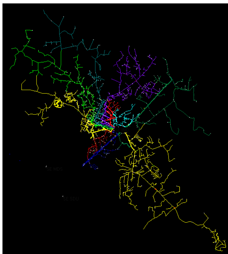
Figura 7 - Mapa Geométrico da subestação Indaiatuba 1 (IND)
