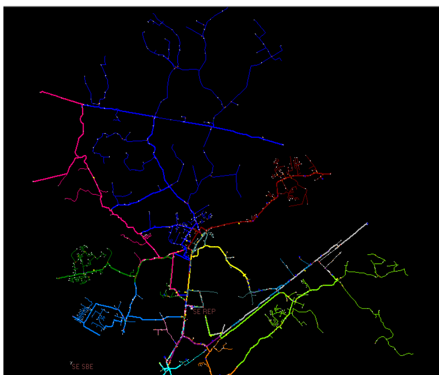
Figura 15 - Mapa Geométrico da subestação Sorocaba2 – Represa (REP)
