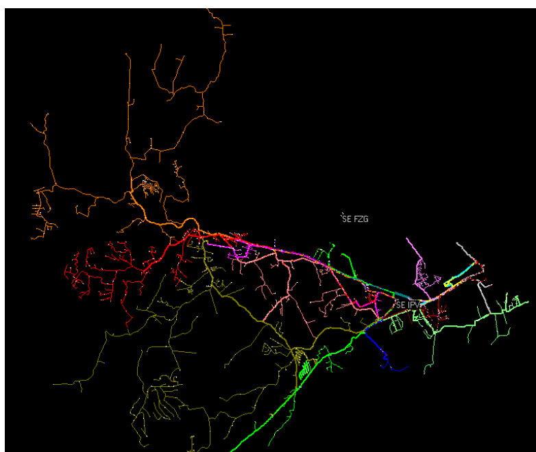
Figura 13 - Mapa Geométrico da subestação Jundiaí 3 – Itupeva (IPV)
