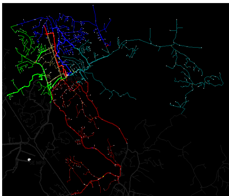
Figura 34 - Mapa Geométrico da subestação Vinhedo 1 (VIN)
