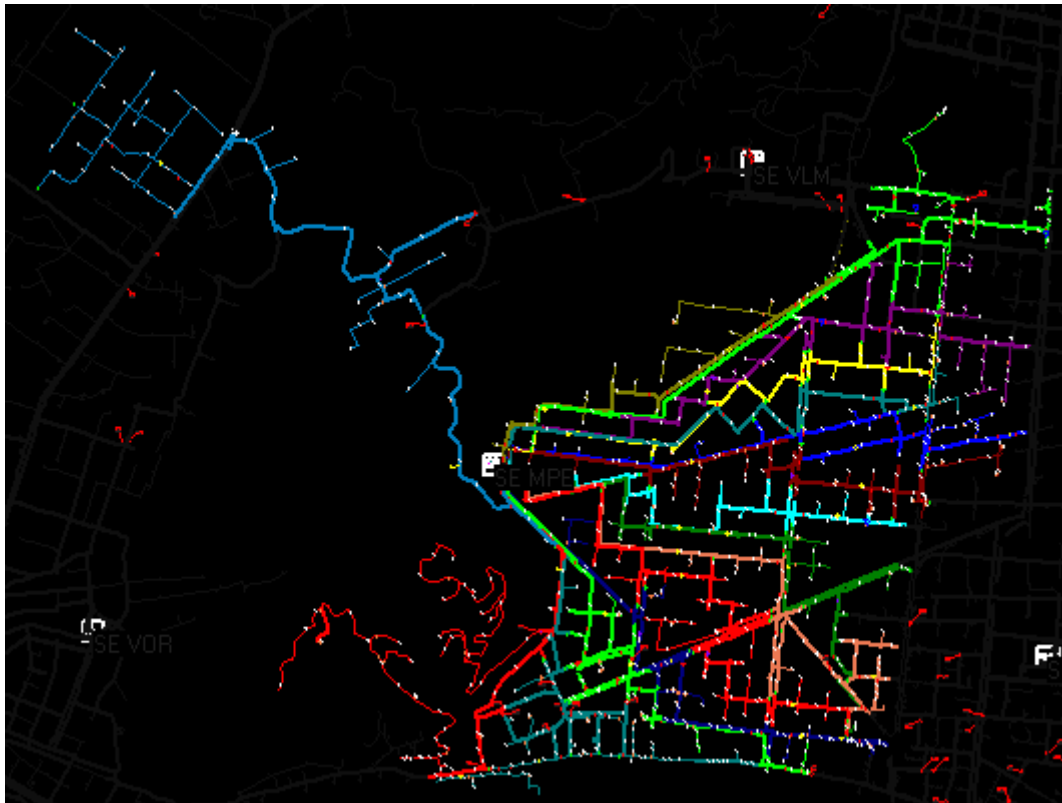
Figura 20 - Mapa Geométrico da subestação Marapé (MPE)
