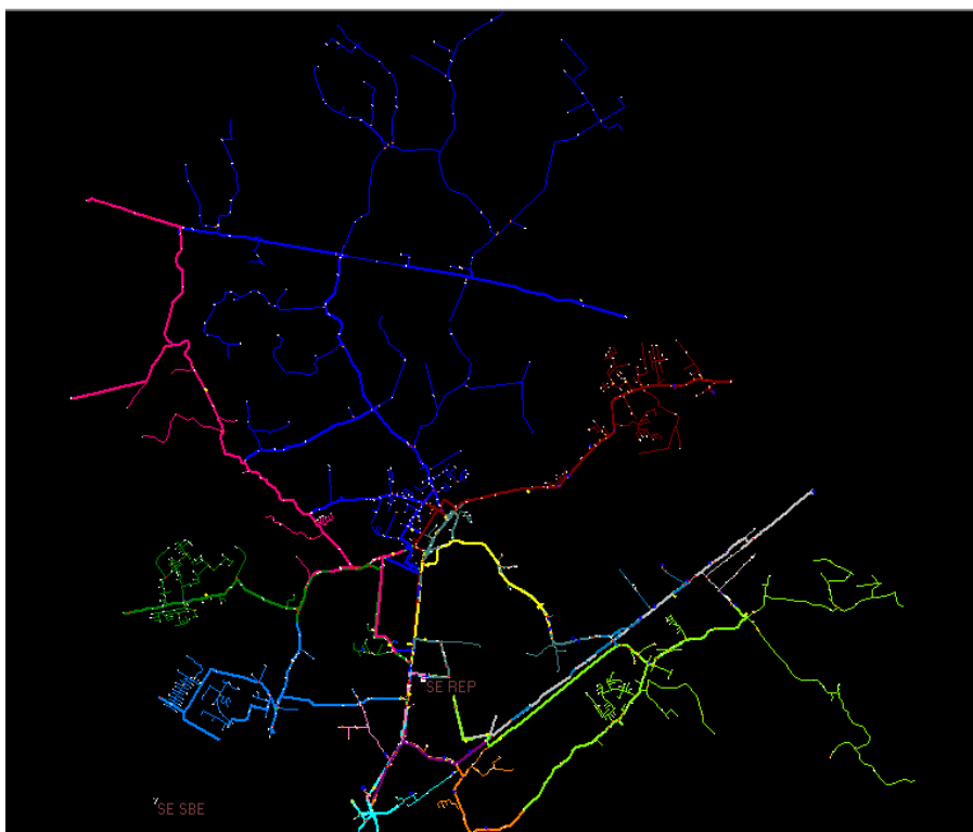
Figura 26 - Mapa Geométrico da subestação Sorocaba2 – Represa (REP)
