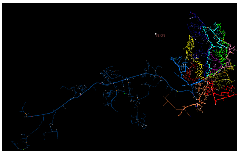
Figura 29 - Mapa Geométrico da subestação Sorocaba 3 – Simus (SIM)
