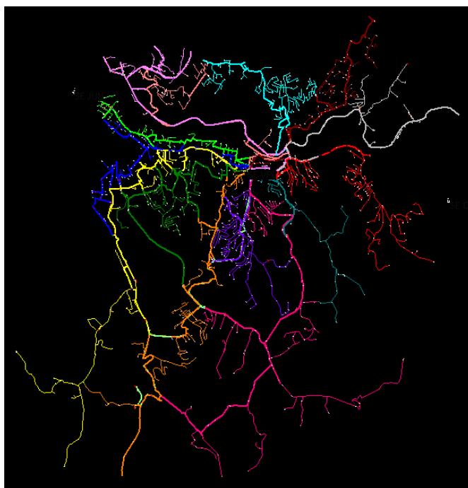
Figura 38 - Mapa Geométrico da subestação Várzea Paulista (VPL)
