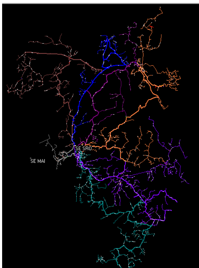
Figura 31 - Mapa Geométrico da subestação São Roque (SRO)
