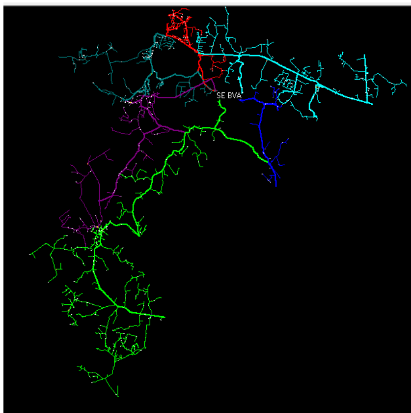
Figura 2 - Mapa Geolétrico da subestação Boituva 1 (BVA)
