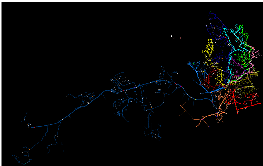
Figura 25 - Mapa Geométrico da subestação Sorocaba 3 – Simus (SIM)
