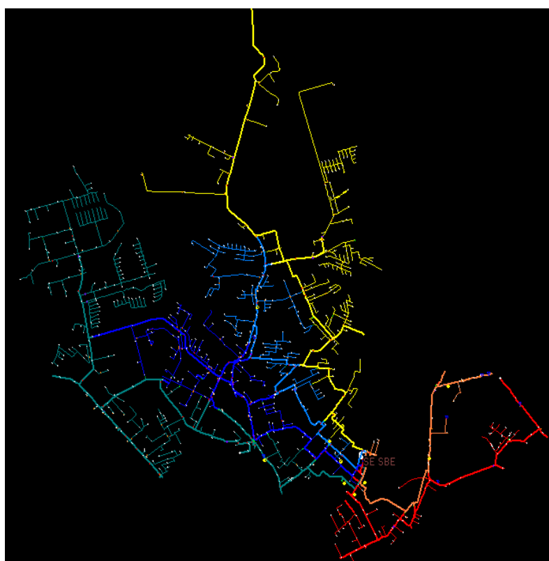
Figura 24 - Mapa Geométrico da subestação Sorocaba 5 - São Bento (SBE)
