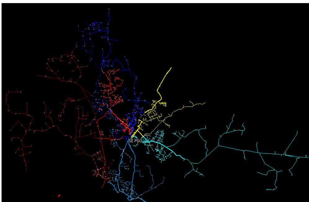
Figura 19 - Mapa Geométrico da subestação Salto 1 – Porto Goes (PGO)
