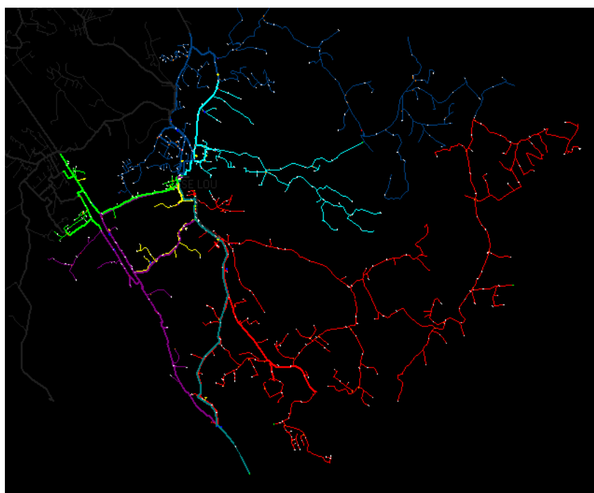
Figura 12 - Mapa Geométrico da subestação Louveira (LOU)
