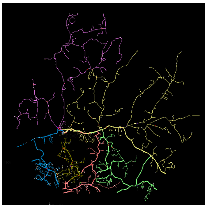
Figura 5 - Mapa Geométrico da subestação Jundiá 5 – Caxambu (CXB)
