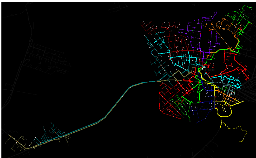
Figura 15 - Mapa Geométrico da subestação São Vicente 2 - Mario Brigidio (MBR)
