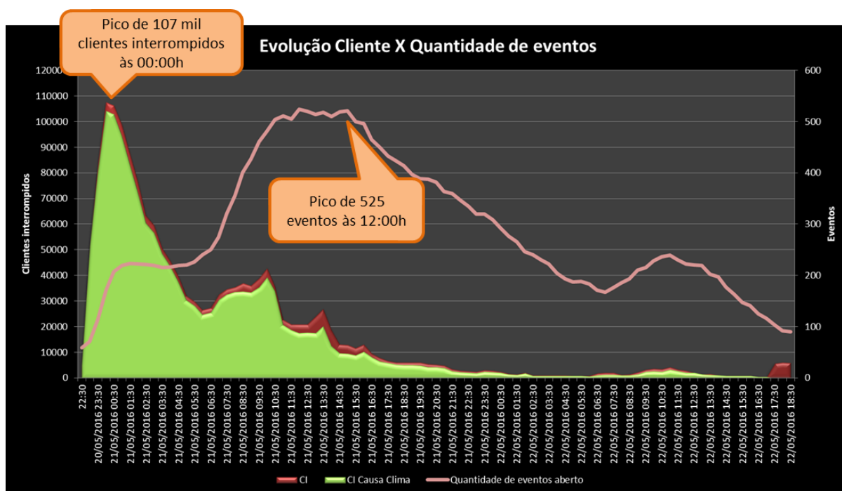
Gráfico 2 – Curva de CI e Ocorrências durante Evento Climático
