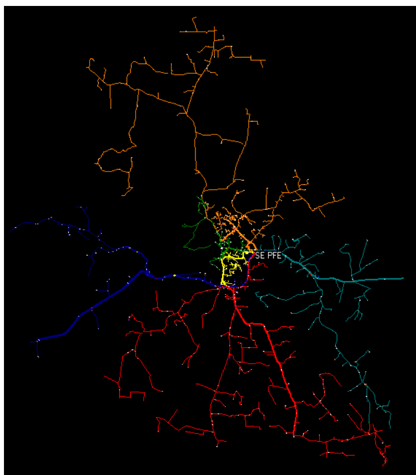
Figura 18 - Mapa Geométrico da subestação Porto Feliz (PFE)
